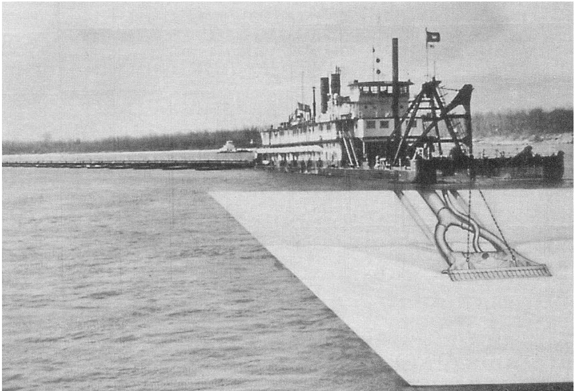
Figura 11.1 – Draga Dustpan mostrando el cabezal de succión
