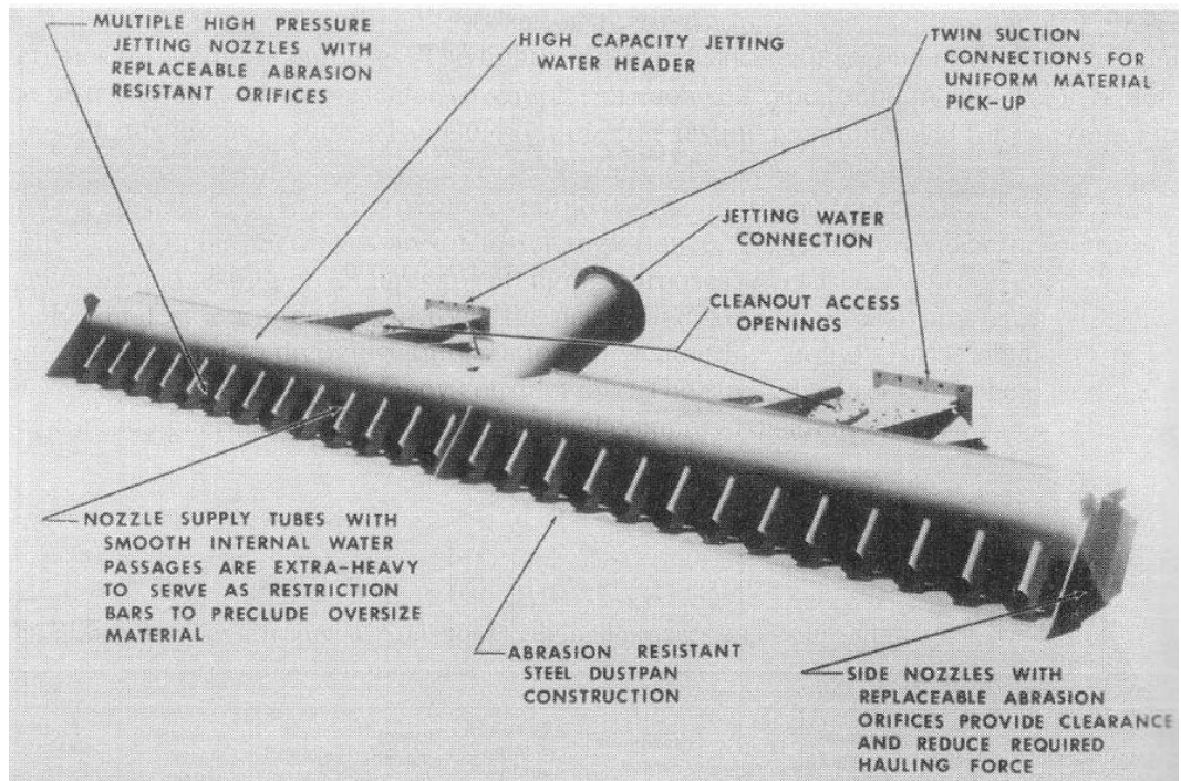
Figura 11.3 – Detalles cabezal de dragado Dustpan
