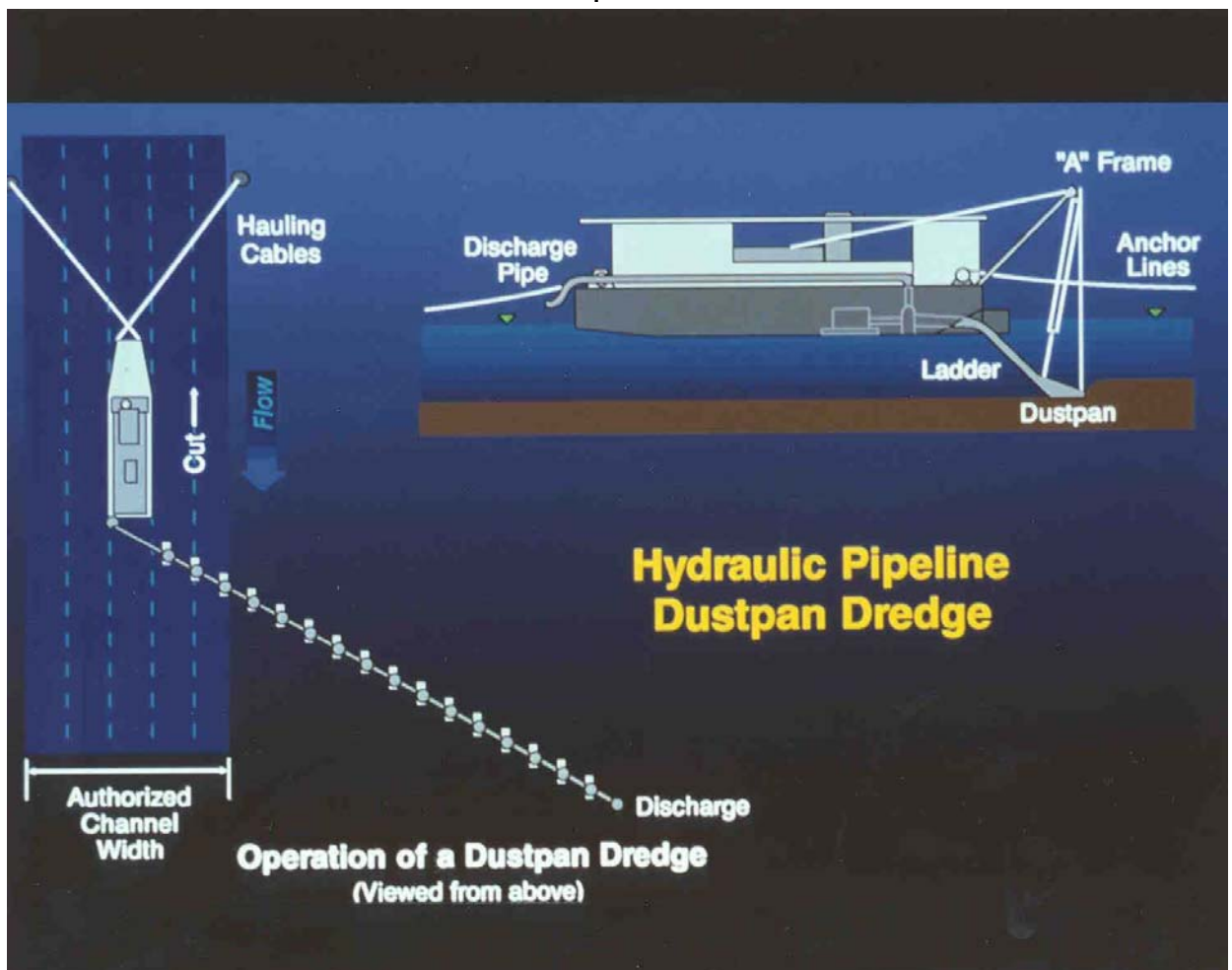
Figura 11.5 – Operación draga Dustpan
