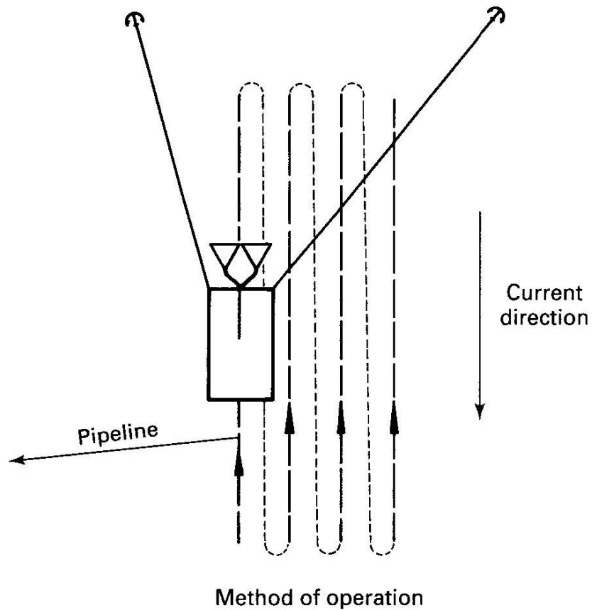
Figura 11.6 – Método de operación
