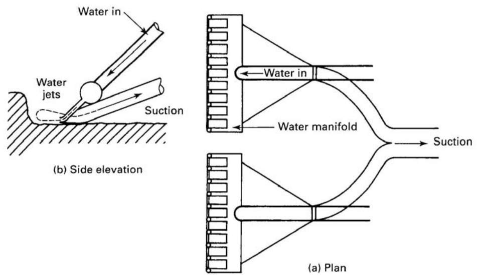
Figura 11.2 – Cabezal de dragado de una draga Dustpan
